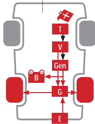
Mischhybrid | Paralleler Zustand
