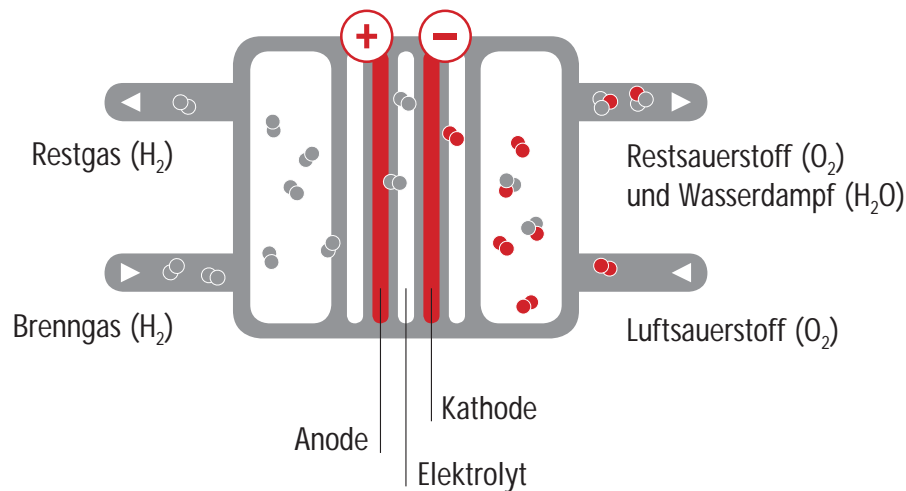
Bauweise einer Brennstoffzelle
