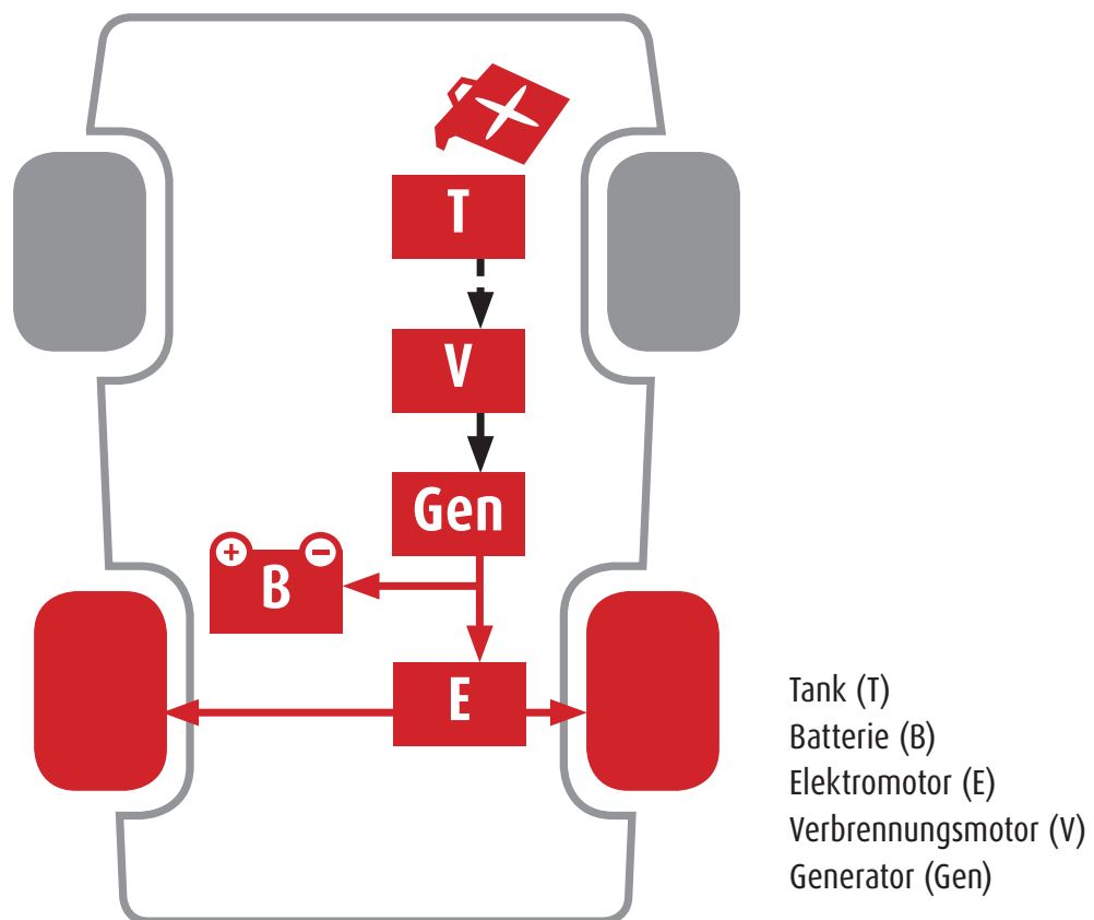
Abbildung eines seriellen Hybrids
