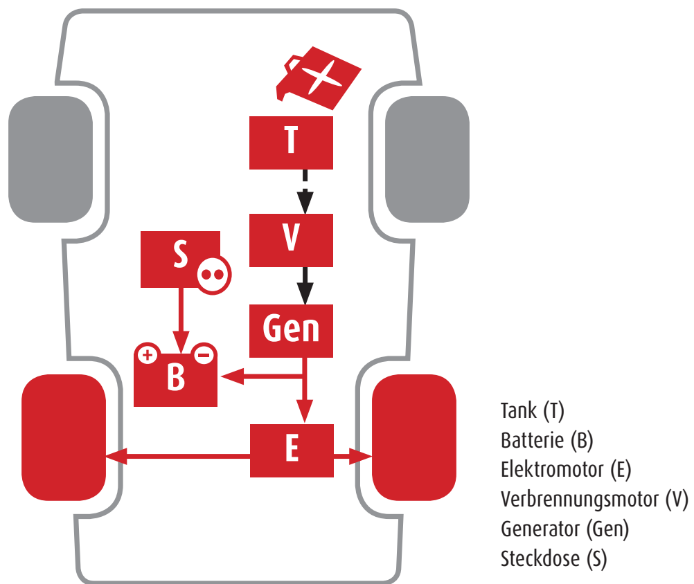
Abbildung eines Plug-In Hybrids
