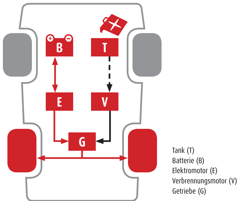
Abbildung eines parallelen Hybrids
